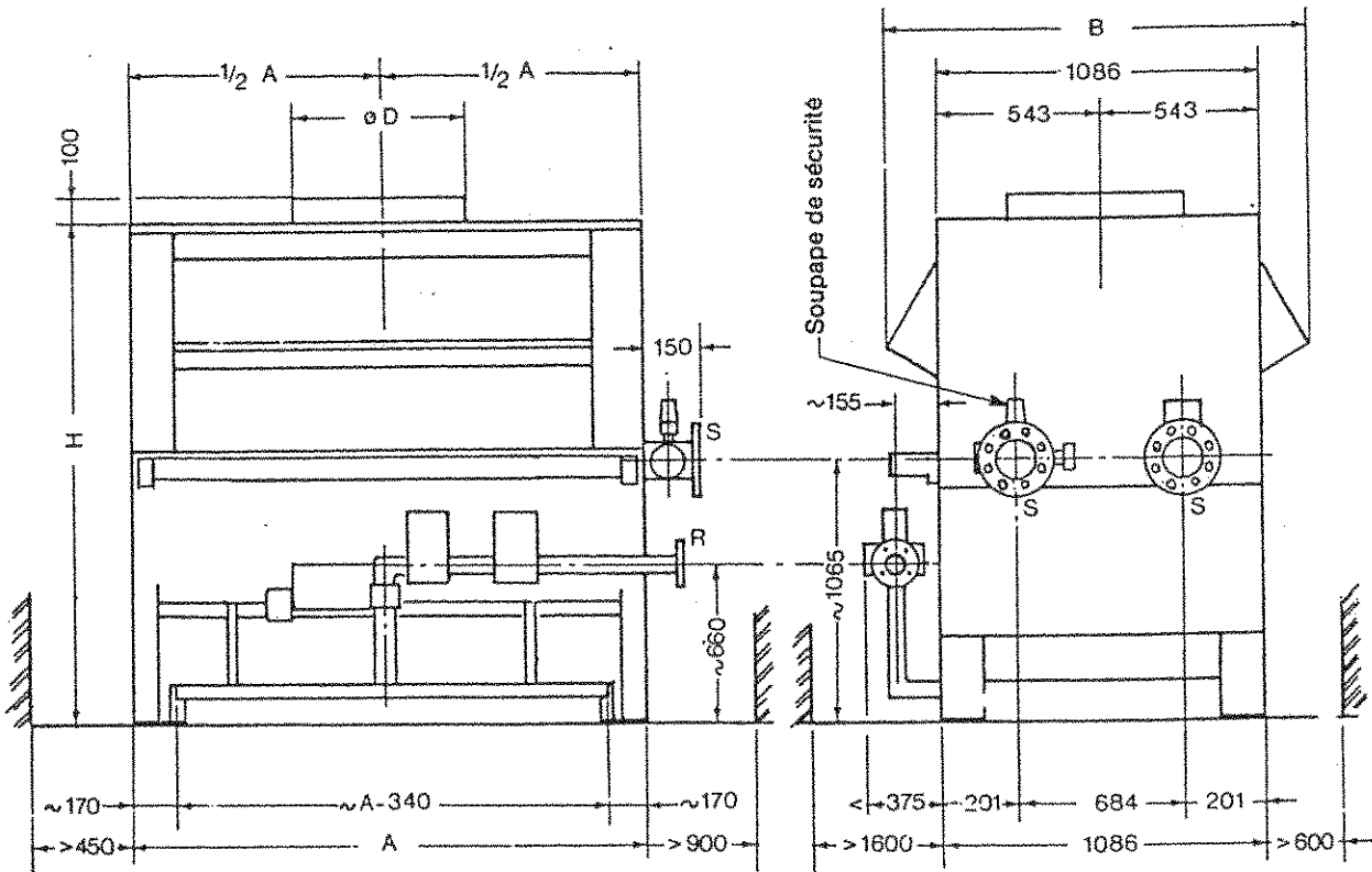
Soupape de sécurité type 132 - 180 : 1 1/4" type 210 - 280 : 1 1/2"
